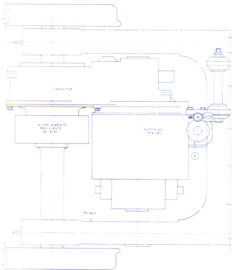
Figura 3 – Detalhe de montagem no truque. O eixo é montado no interior do redutor.
