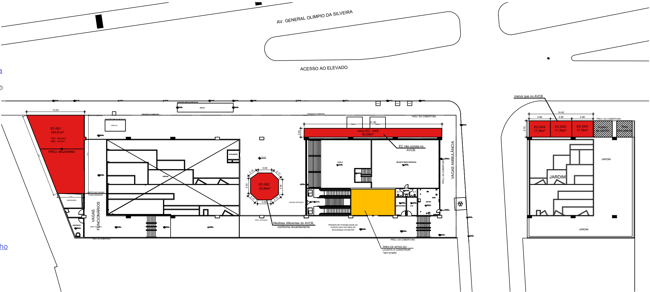
NÍVEL A - ACESSO SEM ESCALA
