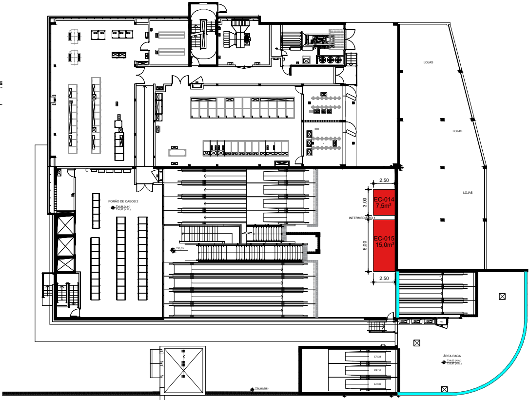
3 PLANTA NÍVEL INTERLIGAÇÃO
